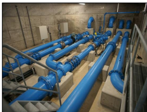
配水塔内配管 P L P φ350～φ450
