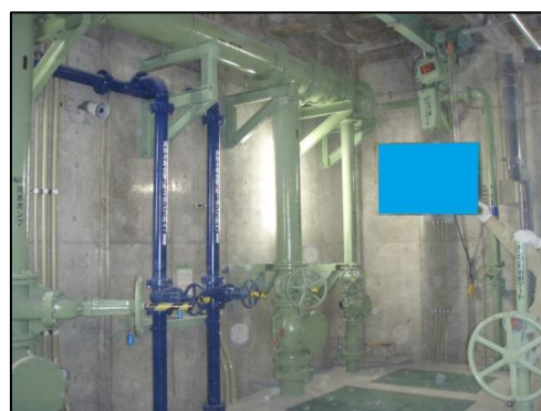
主ポンプ設備（污水ポンプ吸込スクリュース付 污水ポンプ・ポンプ井連絡ゲート手動式鋳鉄製角形）
